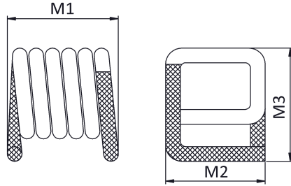
INPAQ TECHNOLOGY CO., LTD. INPAQ TECHNOLOGY CO., LTD. Unit:mm
