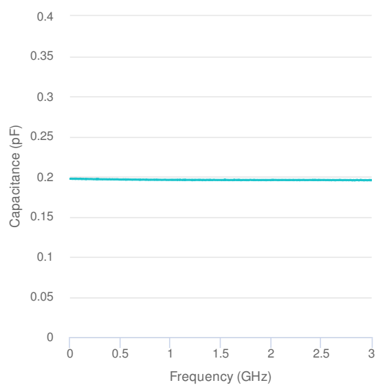
電容頻率曲線
