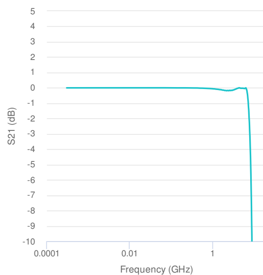
插入損失曲線
