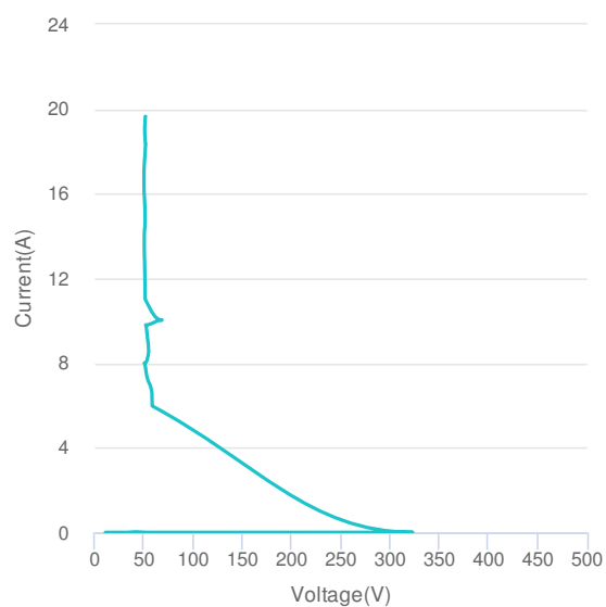
傳輸線脈衝測試曲線
