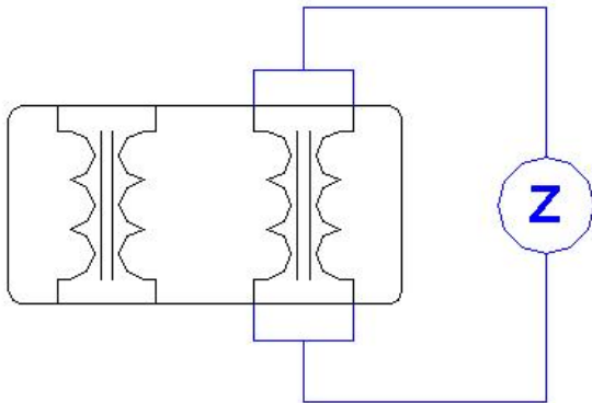
(A):Common mode
